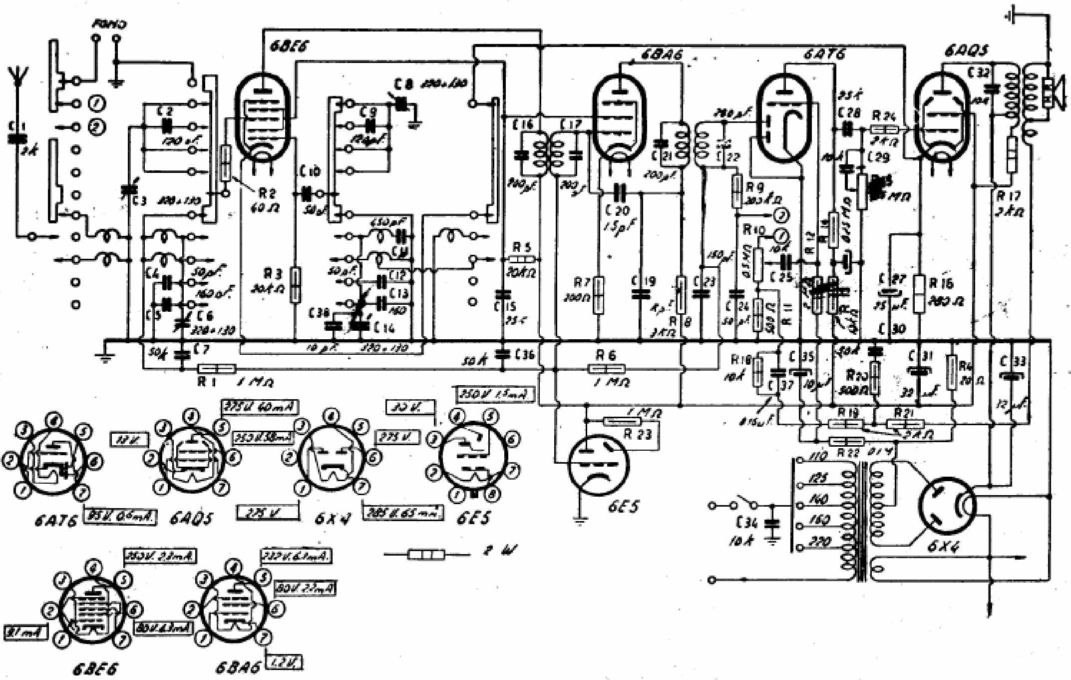
WATT RADIO - Mod. WR 650 IV. Una gamma onde medie, una gamma onde corte e due gamme OC espanse. Media frequenza 470 kc/s. Potenza di uscita indistorta 3 watt.
